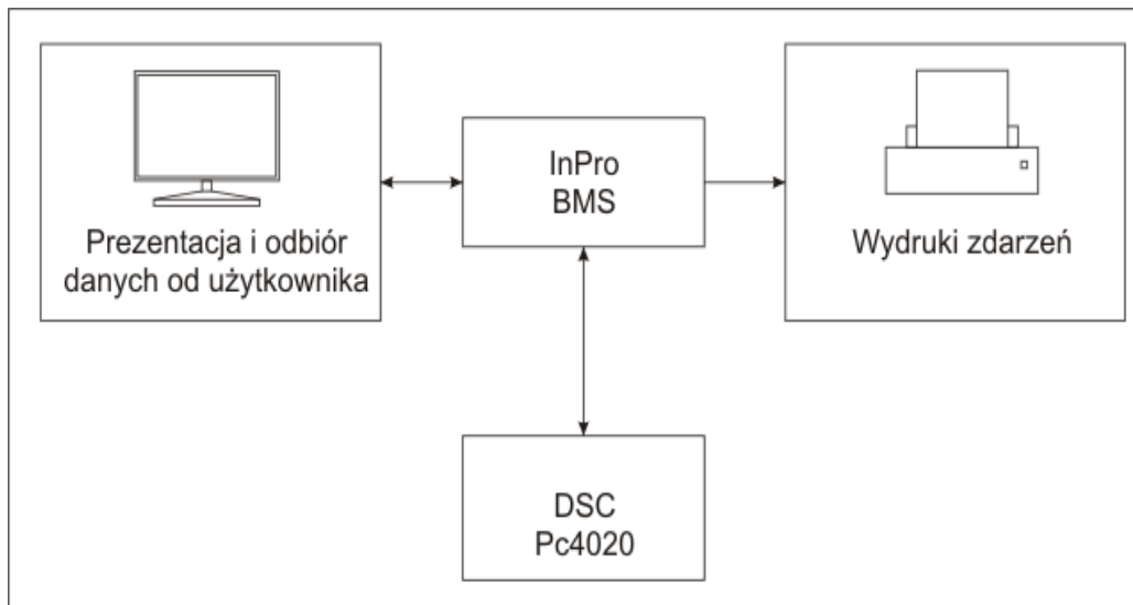
Rys. Przepływ danych w InPro BMS
