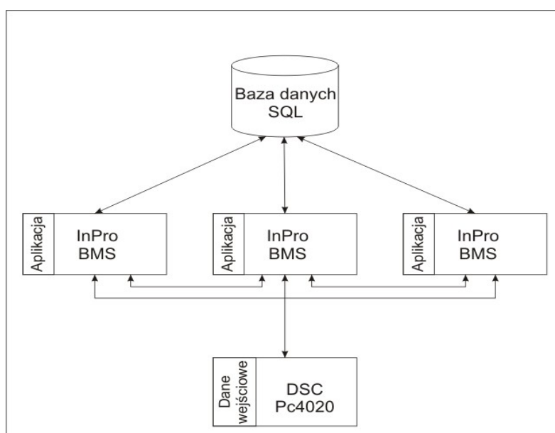
Rys. Struktura oprogramowania InPro BMS.
