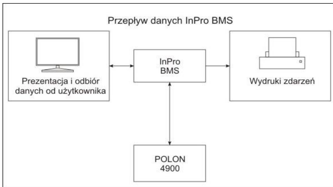
Rys. Przeptyw danych w InPro BMS
