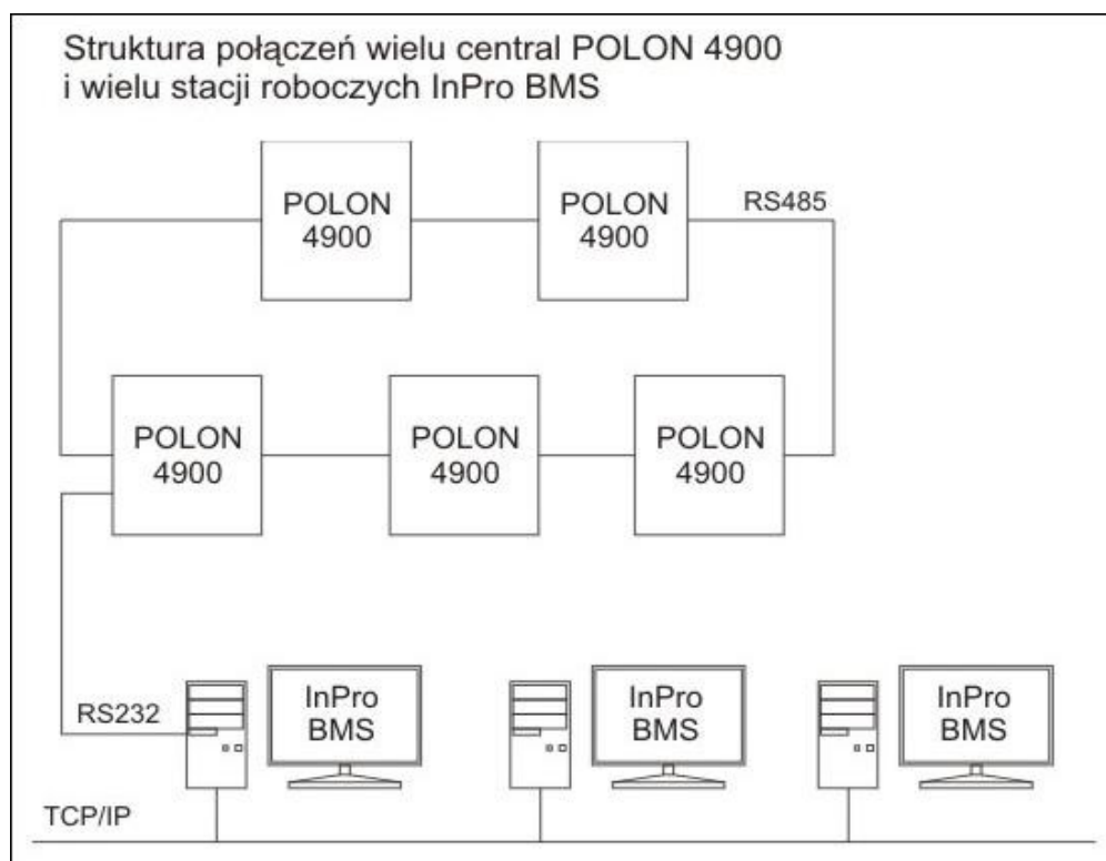
Rys. Struktura połączeń wielu central POLON i wielu stacji roboczych InPro BMS.
