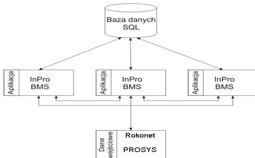
Rys. Struktura oprogramowania InPro BMS.
