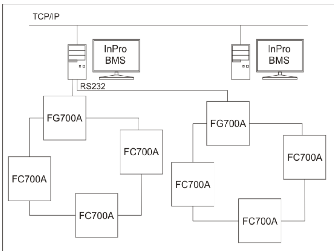
Rys. Połączenie wielu central z InPro BMS.
