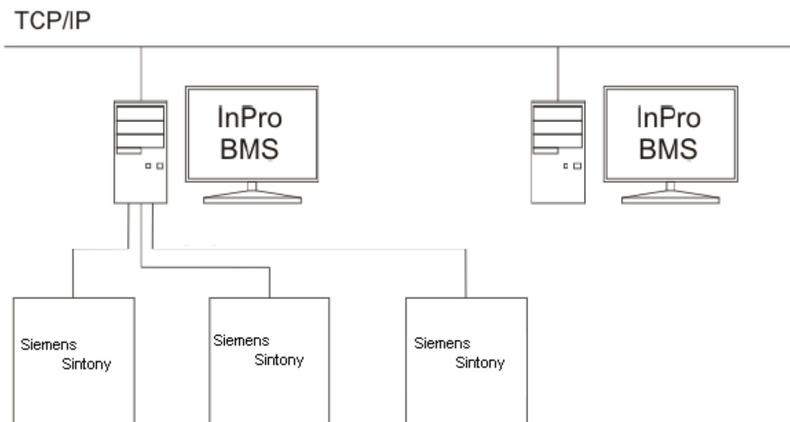
Rys. Struktura połączeń wielu central Siemens SPC i wielu stacji roboczych InPro BMS.
