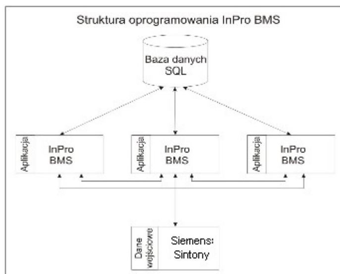
Rys. Struktura oprogramowania InPro BMS.
